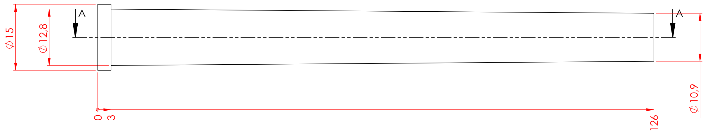
SEZIONE A-A SCALA 2 : 1
