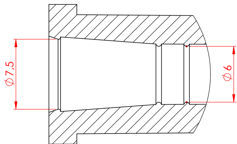
DETTAGLIO B SCALA 4 : 1
